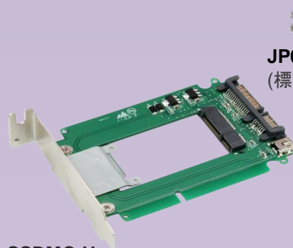
SSDMC-U (USB インターフェース付 SATA-mSATA アダプタ) x1 * ロープロファイル PCIe ブラケット付属
