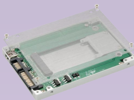
SSDMC-U (USB インターフェース付 2.5 インチ HDD 型 SATA-mSATA アダプタ) x1
