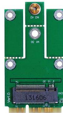
mPCIe Module
