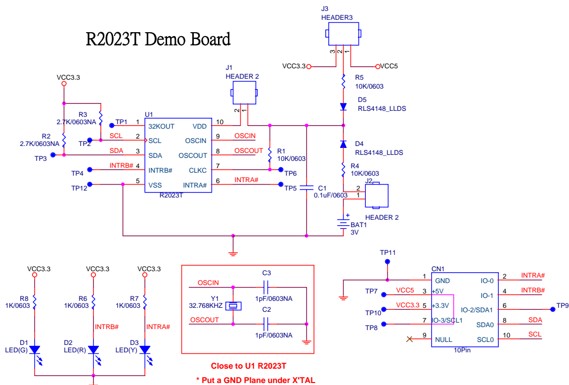
图1 R2023T Demo Board线路
