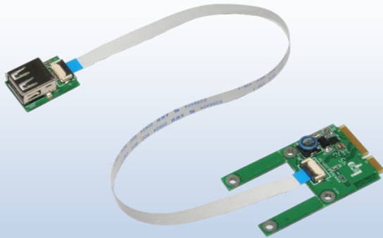
KZ-B34-USB (MiniCard-USB エクステンダ)x1
