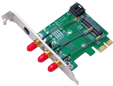
MP2W (無線通信 MiniCard 用 PCIe アダプタ) x1 IPX-RP-SMA ケーブル x3 同梱
