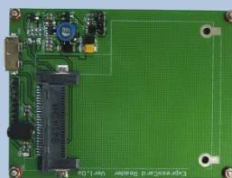
EC03 モジュール (USB3.0-Expresscard 2.0 アダプタ) x1 * モジュールのみ、筐体なし
